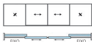
2 folhas + 2 fixos
